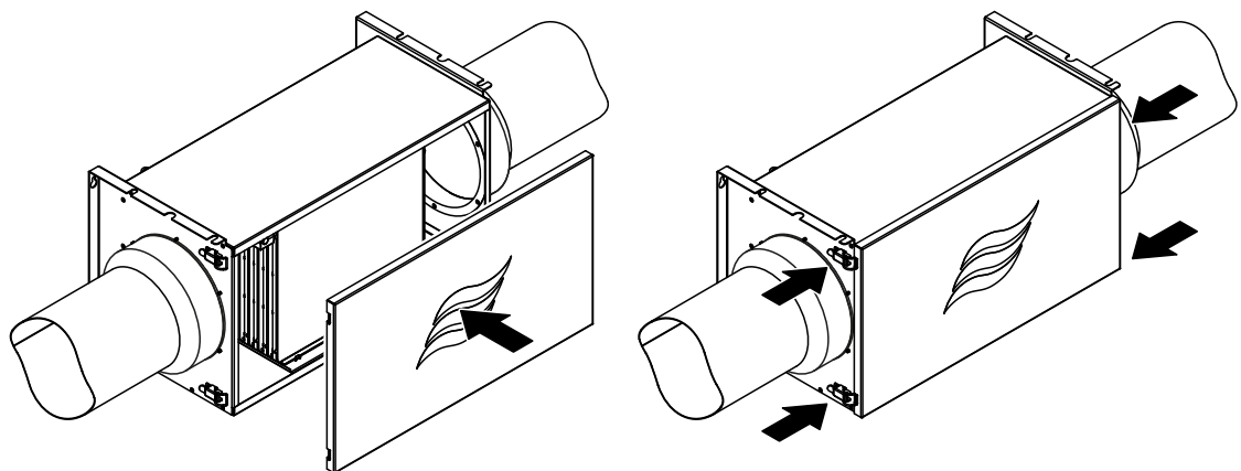
Abb. 19: Befeuchtereinheit schliessen
