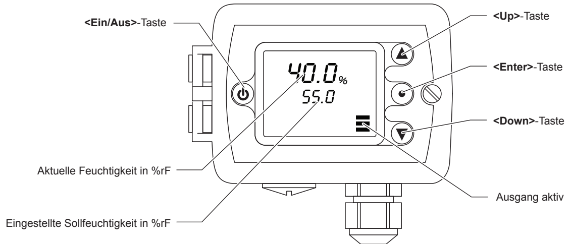
Abb. 10: Bedienelemente Maximalhygrostat
