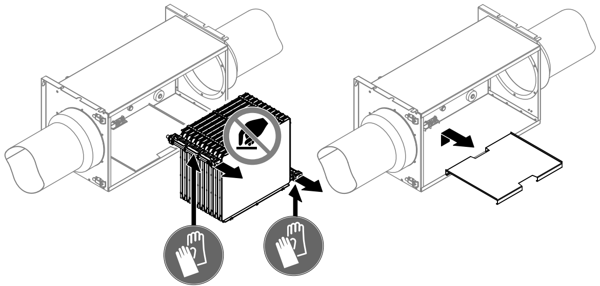
Abb. 21: Befeuchtereinsatz und Bodenblech ausbauen
