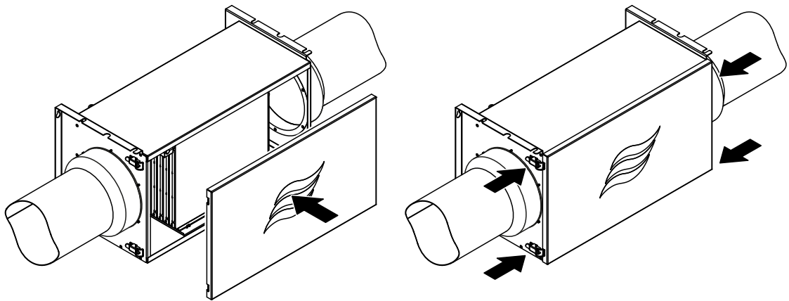
Abb. 25: Befeuchtereinheit schliessen
